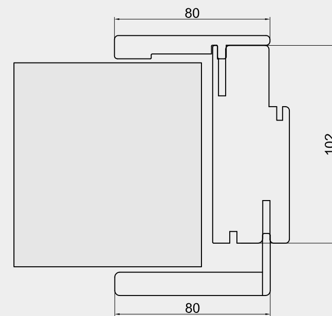
Per muro spesso da 9.5 a 11 cm
