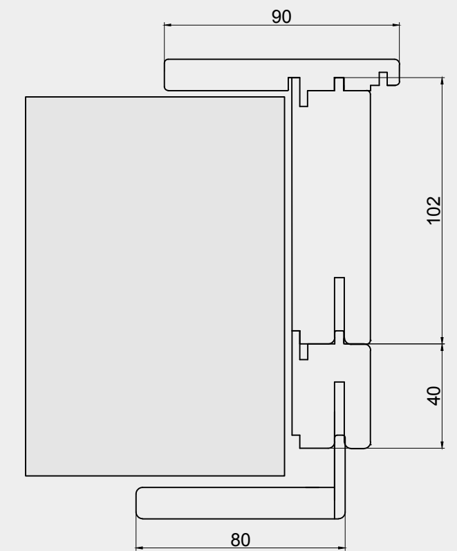
Allargamento per muro spesso da 13.5 a 15 cm Footing for thickness from 13.5 to 15 cm Elargissement pour epaisseur de mur de 13.5 à 15 cm Expansión pared de 13.5 a 15 cm
