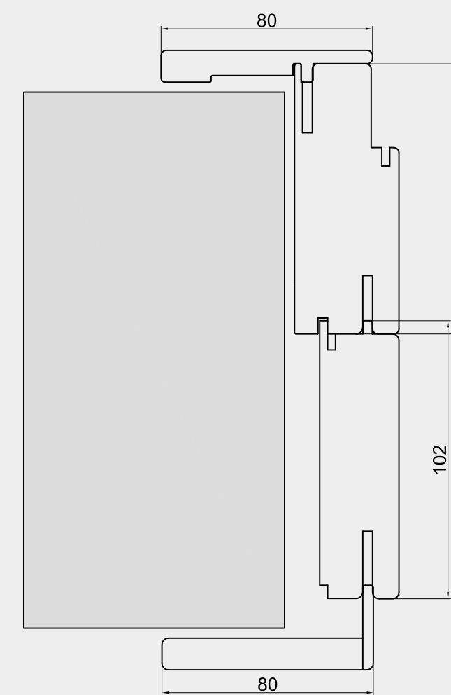
Allargamento per muro spesso da 19.5 a 21 cm
