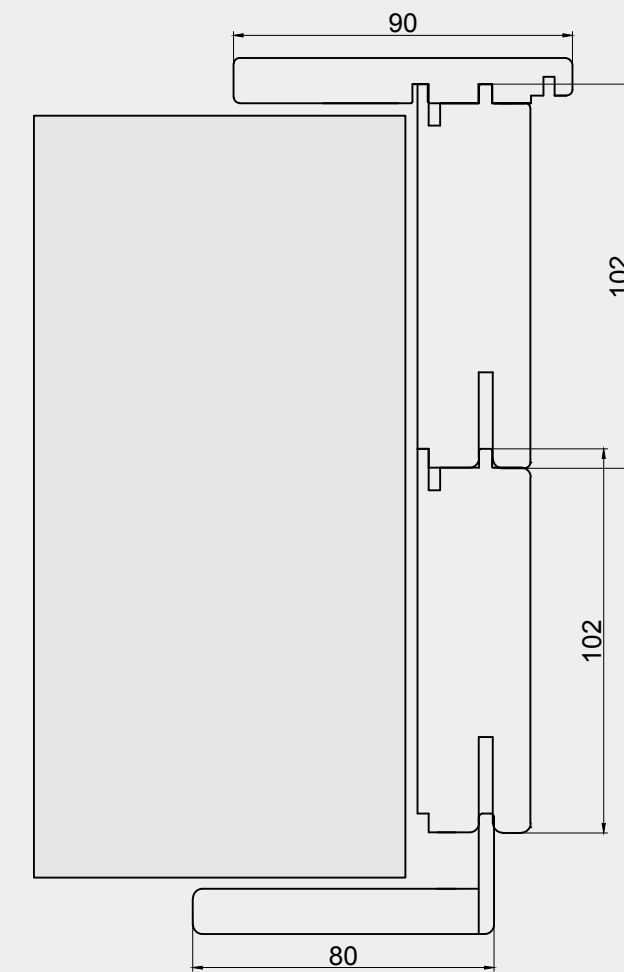
Allargamento per muro spesso da 19.5 a 21 cm Footing for thickness from 19.5 to 21 cm Elargissement pour epaisseur de mur de 19.5 à 21 cm Expansión pared de 19.5 a 21 cm
