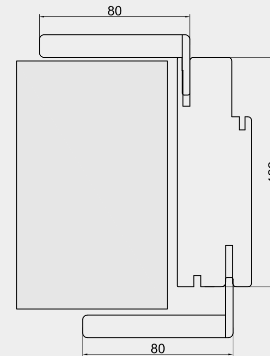
Per muro spesso da 12 a 13.5 cm For thickness from 12 to 13.5 cm Elargissement pour épaisseur de mur de 12 à 13.5 cm Expansión pared de 12 a 13.5 cm
