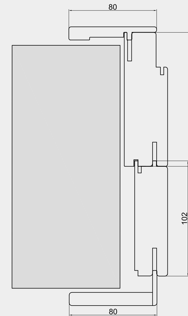
Allargamento per muro spesso da 21.5 a 23 cm
