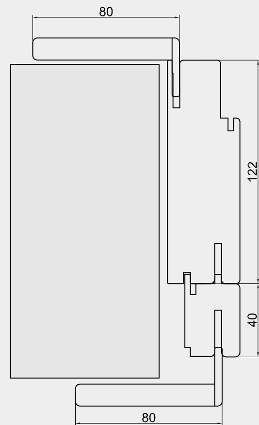
Allargamento per muro spesso da 16 a 17.5 cm Footing for thickness from 16 to 17.5 cm Elargissement pour épaisseur de mur de 16 à 17.5 cm Expansión pared de 16 a 17.5 cm
