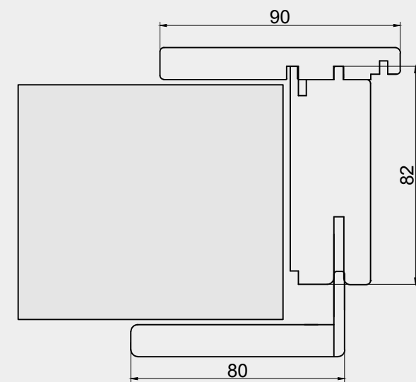
Per muro spesso da 7.5 a 9 cm For thickness from 7.5 to 9 cm Elargissement pour epaisseur de mur de 7.5 à 9 cm Expansión pared de 7.5 a 9 cm
