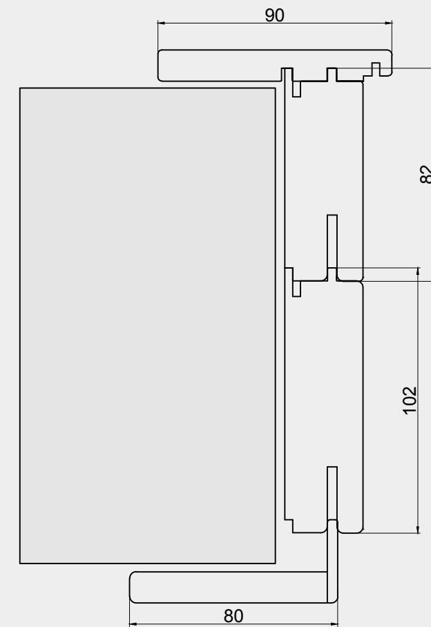
Allargamento per muro spesso da 17.5 a 19 cm Footing for thickness from 17.5 to 19 cm Elargissement pour epaisseur de mur de 17.5 à 19cm Expansión pared de 17.5 a 19 cm
