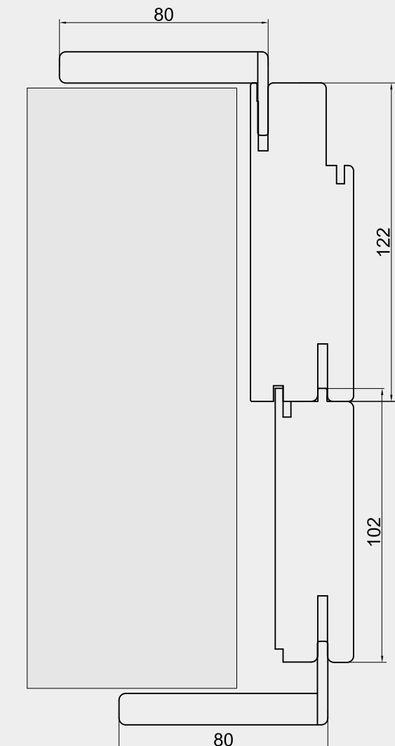
Allargamento per muro spesso da 22 a 23.5 cm Footing for thickness from 22 to 23.5 cm Elargissement pour épaisseur de mur de 22 à 23.5 cm Expansión pared de 22 a 23.5 cm
