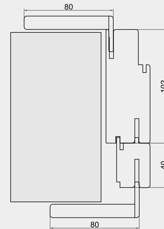
Allargamento per muro spesso da 14 a 15.5 cm Footing for thickness from 14 to 15.5 cm Elargissement pour épaisseur de mur de 14 à 15.5 cm Expansión pared de 14 a 15.5 cm
