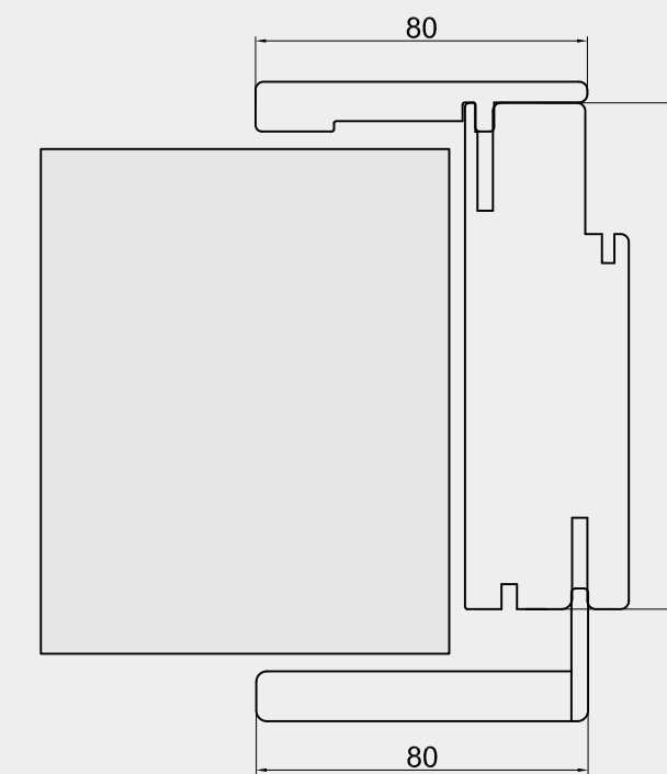
Per muro spesso da 11.5 a 13 cm
