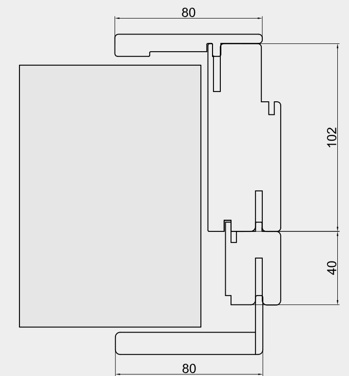
Allargamento per muro spesso da 13.5 a 15 cm
