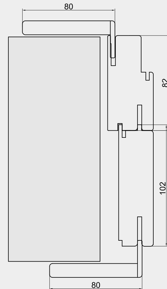
Allargamento per muro spesso da 18 a 19.5 cm Footing for thickness from 18 to 19.5 cm Elargissement pour épaisseur de mur de 18 à 19.5 cm Expansión pared de 18 a 19.5 cm
