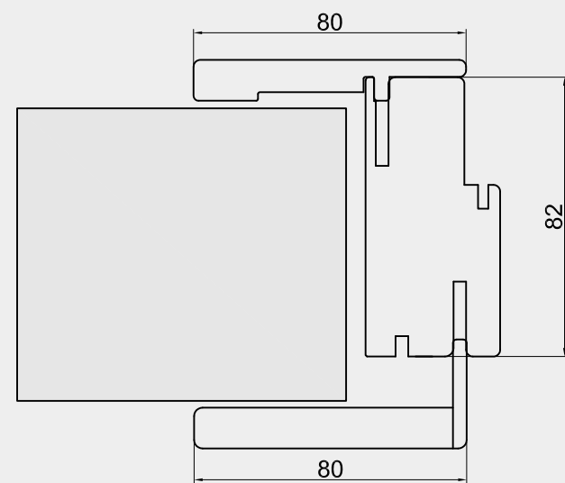
Per muro spesso da 7.5 a 9 cm
