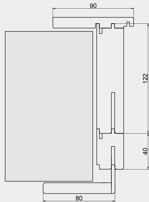
Allargamento per muro spesso da 15.5 a 17 cm Footing for thickness from 15.5 to 17 cm Elargissement pour epaisseur de mur de 15.5 à 17 cm Expansión pared de 15.5 a 17 cm
