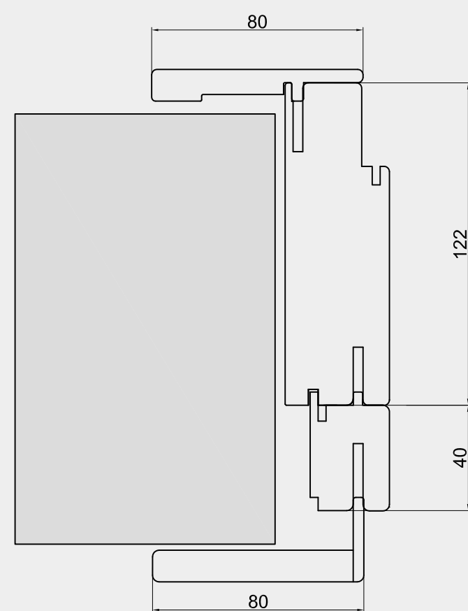
Allargamento per muro spesso da 15.5 a 17 cm
