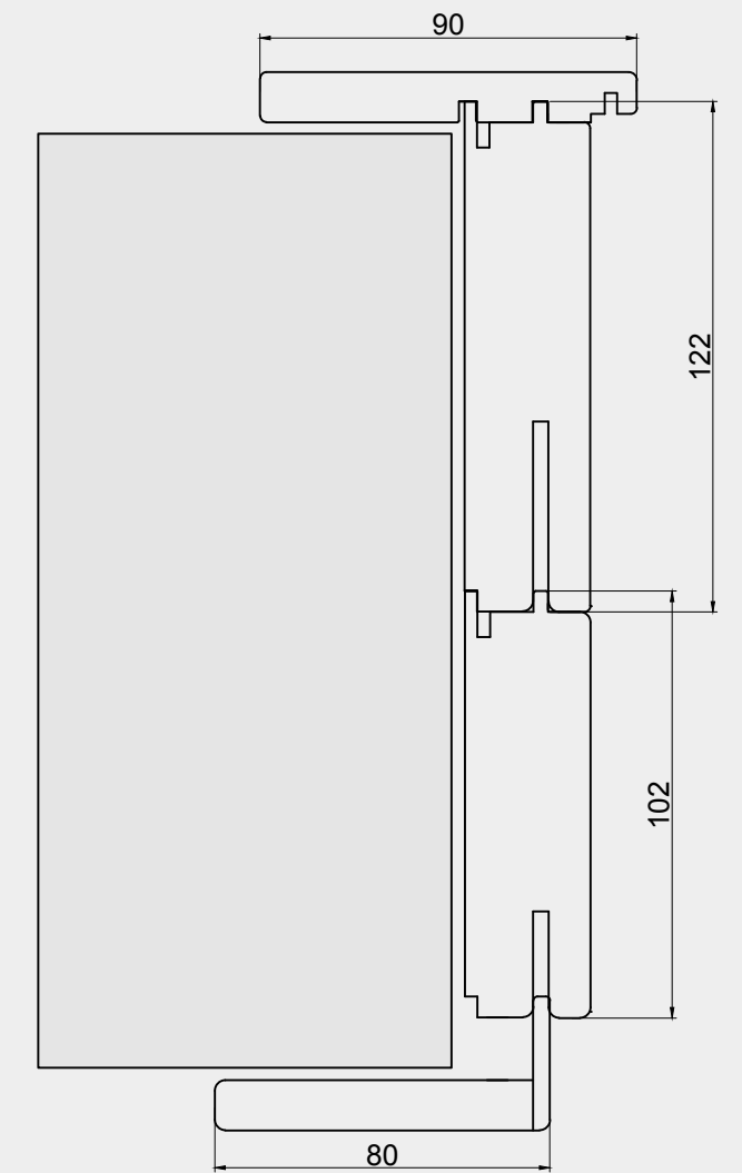
Allargamento per muro spesso da 21.5 a 23 cm Footing for thickness from 21.5 to 23 cm Elargissement pour epaisseur de mur de 21.5 à 23 cm Expansión pared de 21.5 a 23 cm
