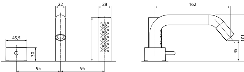
RUBINETTERIA BORDO VASCA (per Stile) con cartuccia di miscelazione progressiva, doccetta di servizio design Marco Pellici
