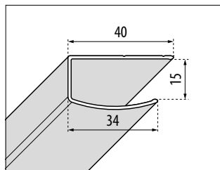
A MURO - FREE 2
