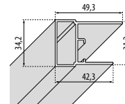
KUADRA 2.0 H 200 cm In sostituzione del profilo a muro +15 mm
