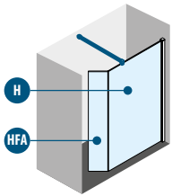
KUADRA H KUADRA HFA BARRA DI SOSTEGNO (in dotazione)
