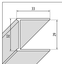
A MURO per Opera FH
