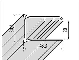
A MURO - FREE 1
