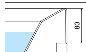
BORDO ALTO - 8 CM
