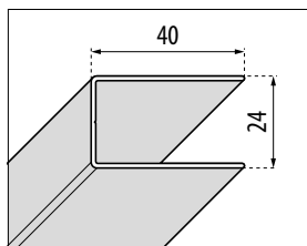
A MURO R - PH+F - A - 3PH
