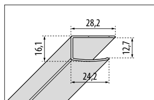
A MURO RIVIERA R
