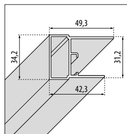
COMPENSAZIONE per tutti i modelli
