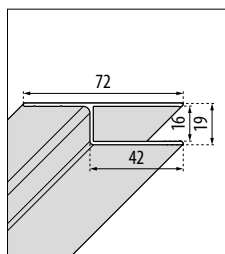
A MURO profilo a muro laterale tutti i modelli
