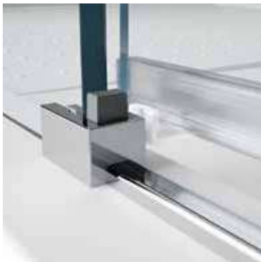
◀ Sistema di sgancio ante scorrevoli per una facile pulizia
